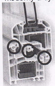
- systém so stredovým tesnením - 3 tesnenia v profile
